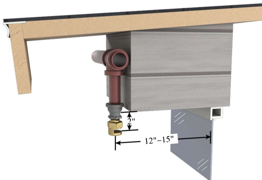
C-1 型水幕喷头安装示意图
