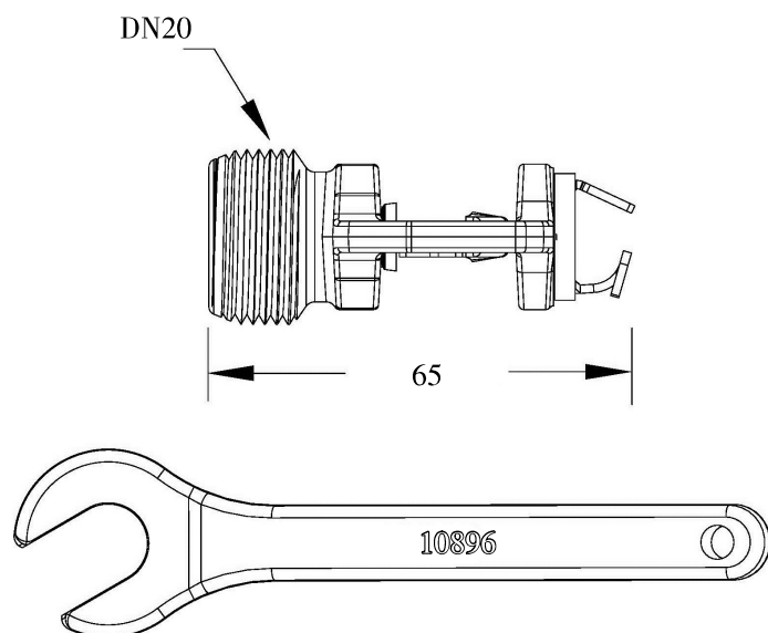
专用扳手型号: 10896W/B
