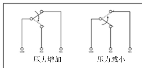
PS10A SPDT 接点动作情况
