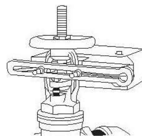
图一 1/2"(15mm)至 2-1/2"(65mm)小阀门安装图
