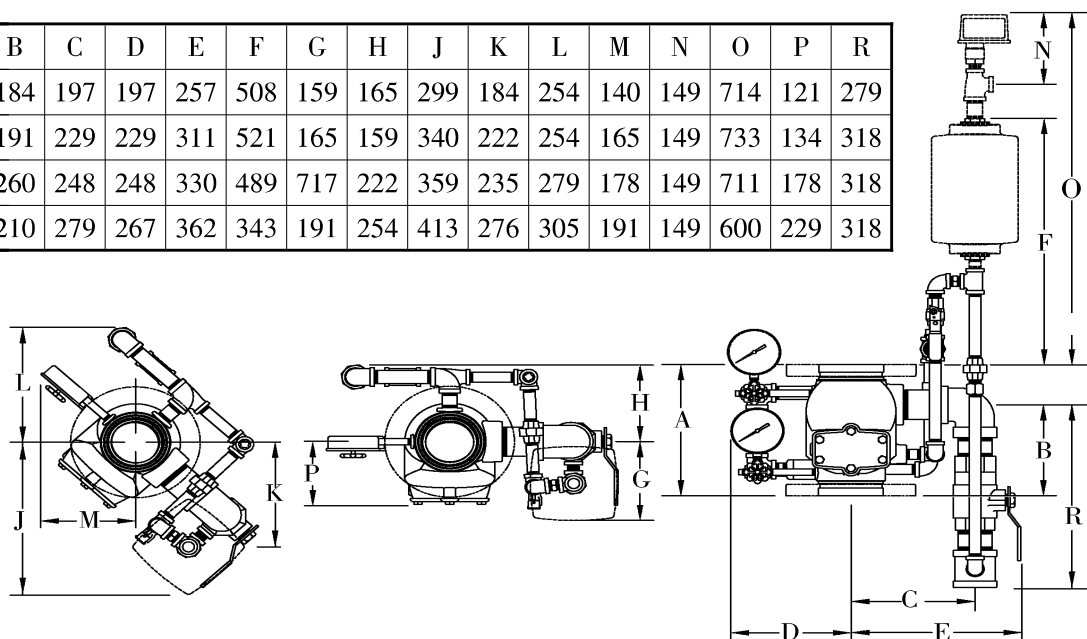
J-1 型垂直安装湿式报警阀(含阀体、配管、延时器、压力开关)
